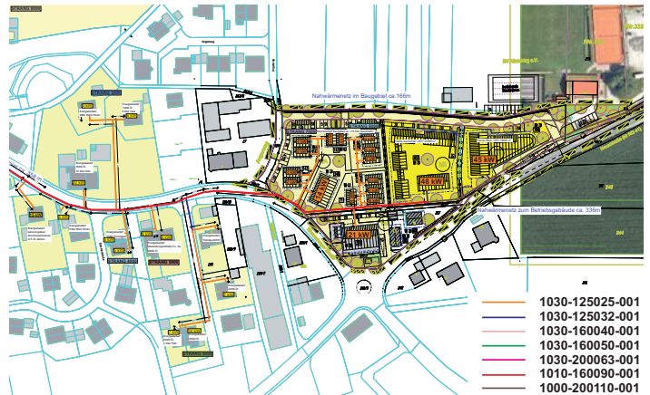
Die bisherige Planung der Fernwärmeleitung (braun,rot,orange) umfasst das neue Baugebiet sowie Anlieger entlang der Wasserburger Straße. Weitere Anschlussgebiete sind möglich.
